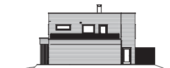
Fasade mot vest
